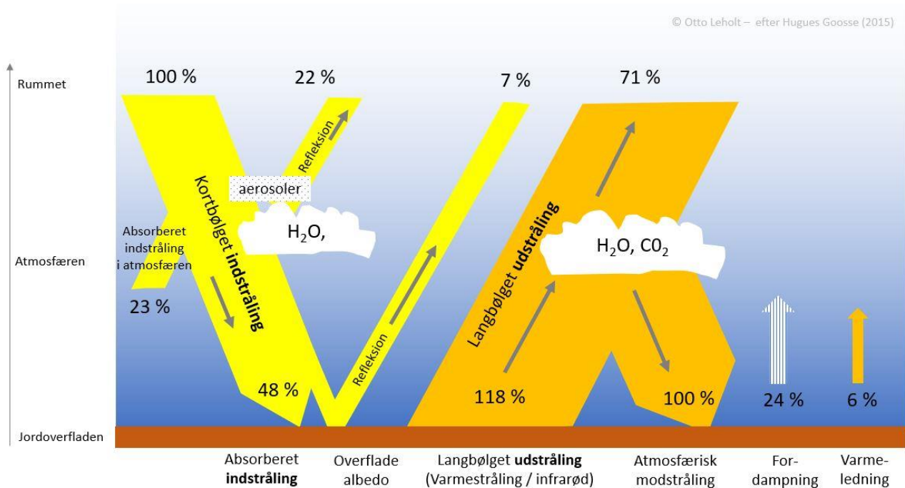
Figur 1: Model over atmosfærens strålingsbalance
