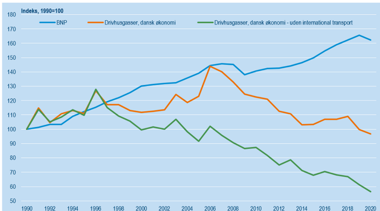
Figur 6: Danmarks udledning af DRIVHUSGASSER 1990-2020
