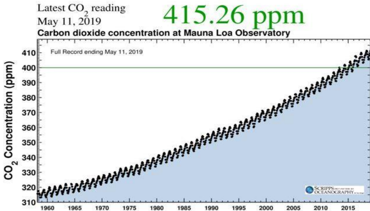
Figur 4: Keeling-kurven med atmosfærens CO 2 koncentration 1958-2019
