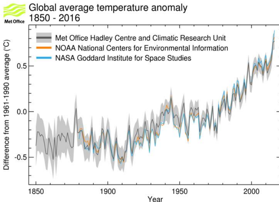
Figur 2: Afvigelser i den globale gennemsnitstemperatur i forhold til referenceperioden (1961-90)
