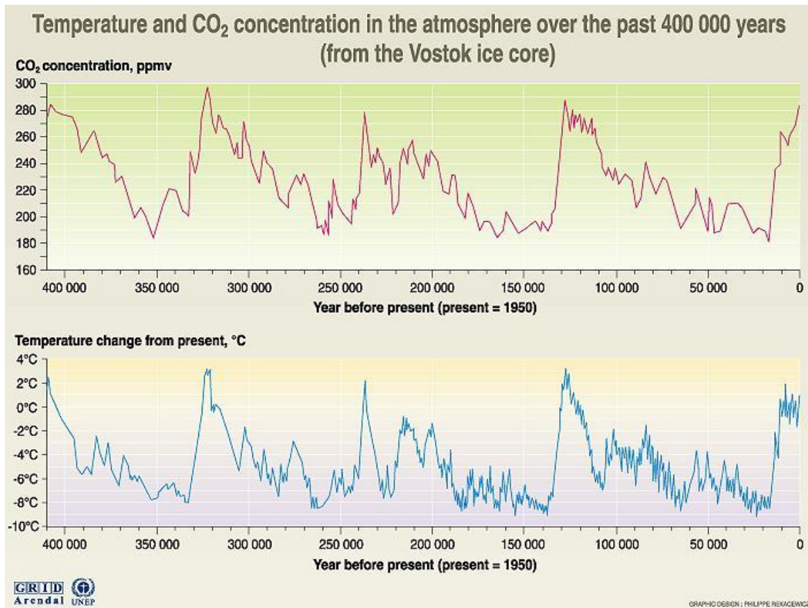
Figur 3: Co2 koncentration og temperaturafvigelser i forhold til 1950 gennem 400.000 år
